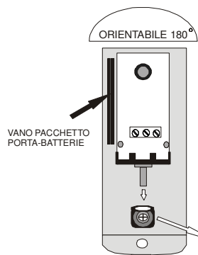
VITE DI BLOCCO ROTAZIONE / ROTATING BLOCK SCREW (VITE IN DOTAZIONE)
